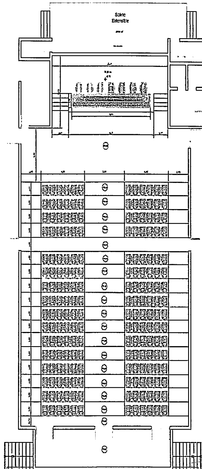
PLAN D'AMEUBLEMENT
